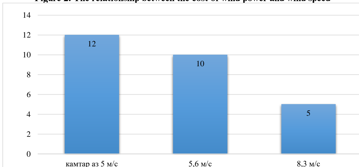
Расми 2. Муносибати байни хароҷоти неруи барқӣ истиҳсолшавандаи бодӣ ва суръати бодӣ Figure 2. The relationship between the cost of wind power and wind speed
