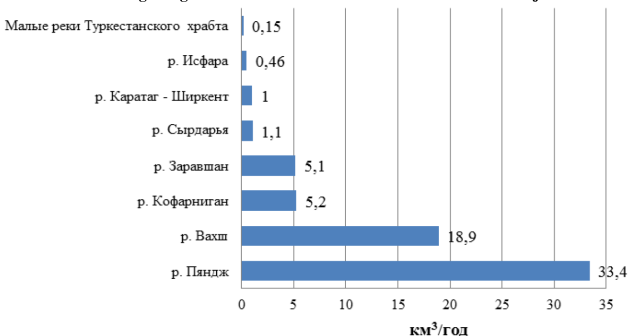
Рис. 1. Среднегодовое количество стока по бассейнам основных рек Таджикистана Rice. 1. Average long-term runoff in the basins of the main rivers of Tajikistan
