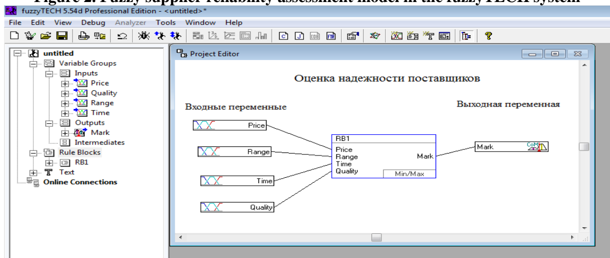
Рисунок 2. Нечеткая модель оценки надежности поставщика в системе fuzzyTECH Figure 2. Fuzzy supplier reliability assessment model in the fuzzyTECH system
