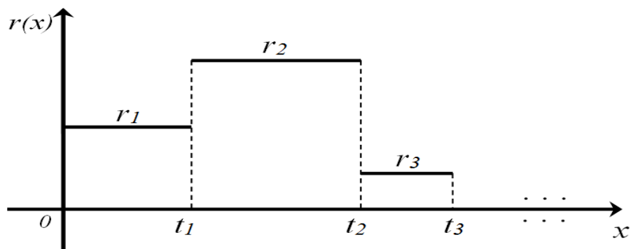
Рис.1. Кусочно-постоянная интенсивность фактора риска Fig. 1. Piece-wise constant intensity of the risk factor
