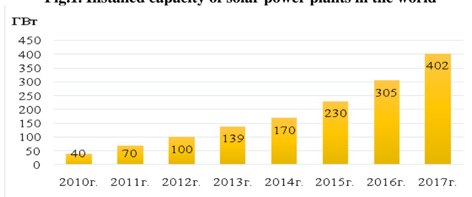
Рис.1. Установленная мощность солнечных электростанций в мире Fig.1. Installed capacity of solar power plants in the world
